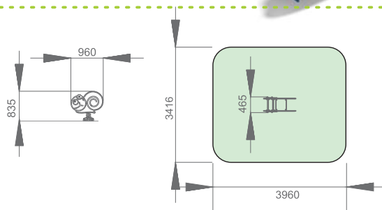
Spring toy «Caterpillar»
