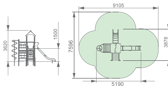
Playground complex «Tower»
