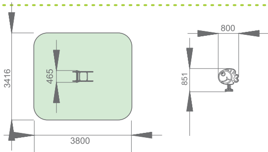
Spring toy «Early bird»
