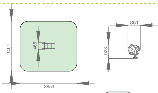
Spring toy «Caterpillar»
