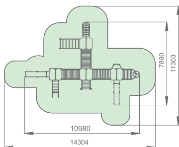
Playground complex «Fortress»
