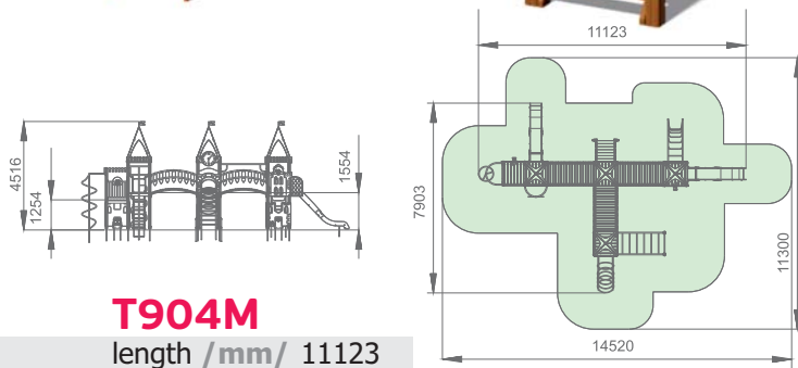
Playground complex «Fortress»-M»
