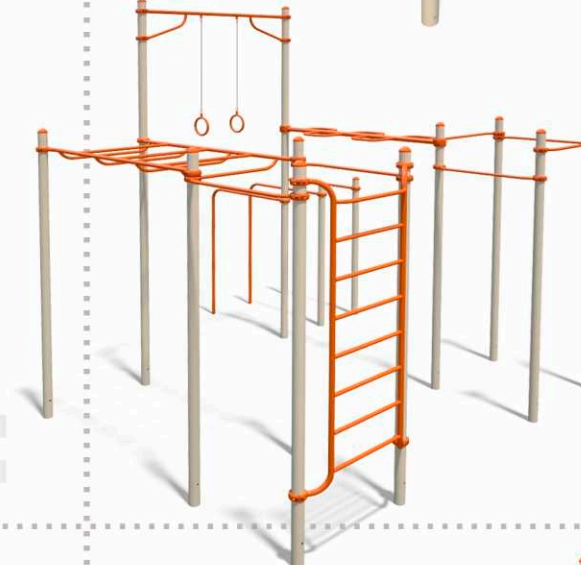
S831.4 length /mm/ 4862 width /mm/ 4557 height /mm/ 4127 weight /kg/ 565
