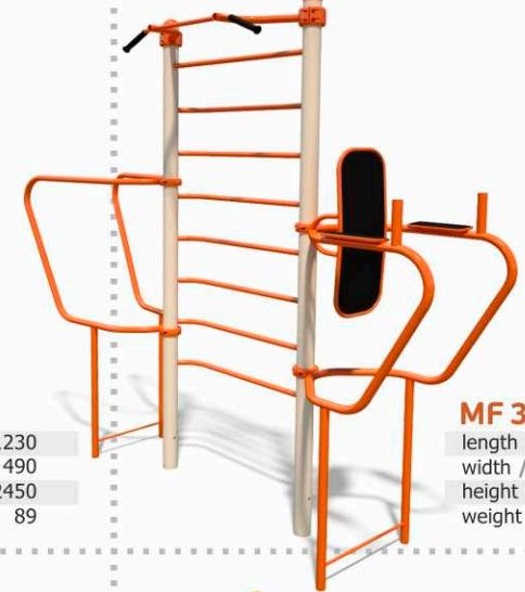
MF3.6 length /mm/ 3259 width /mm/ 2549 height /mm/ 2526 weight /kg/ 198
